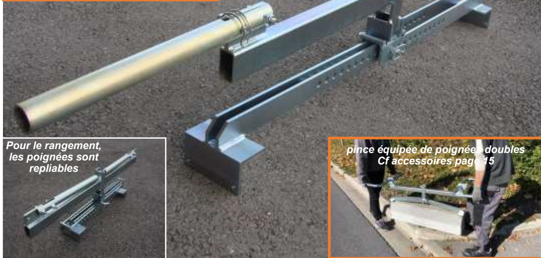
L'ouverture de la pince réf. 9948 est réglable de 50cm à 1.20m
